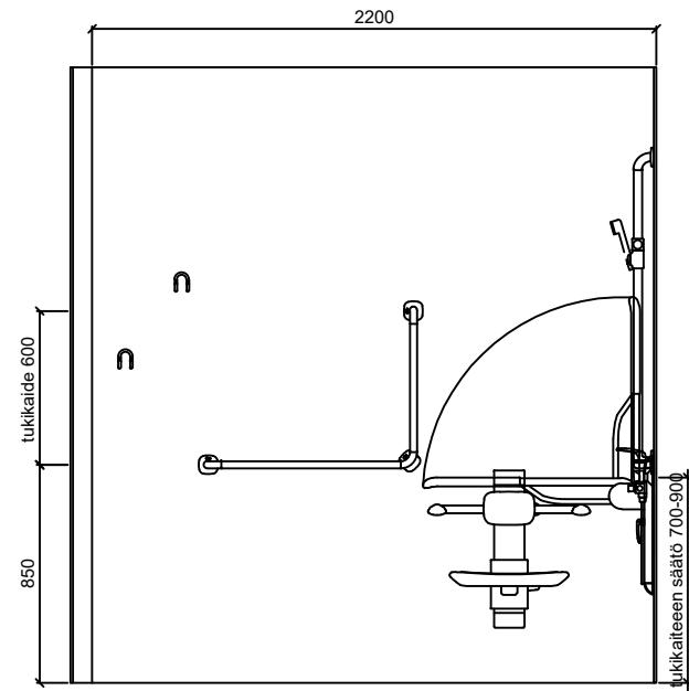
SEINÄKAAVIO C Gaius Sense 2XL
