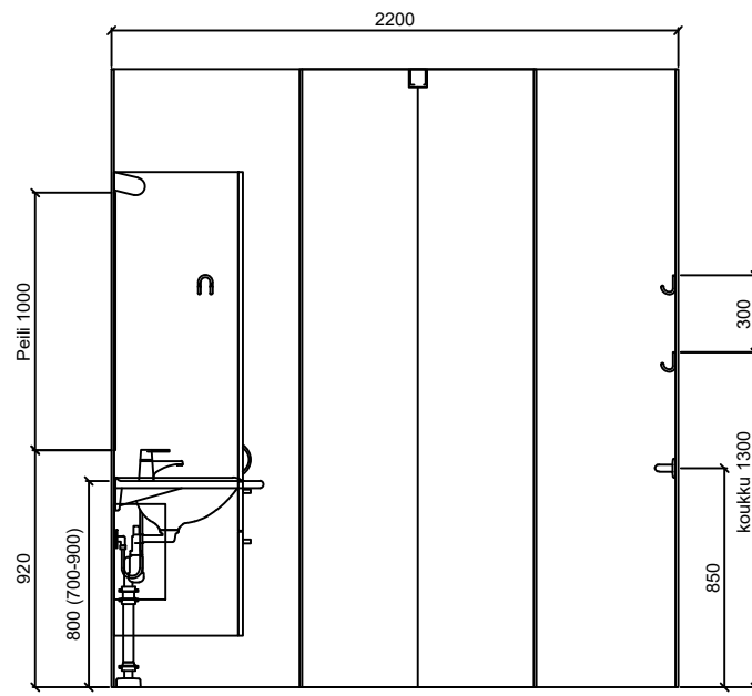
SEINÄKAAVIO B Gaius Sense 2XL
