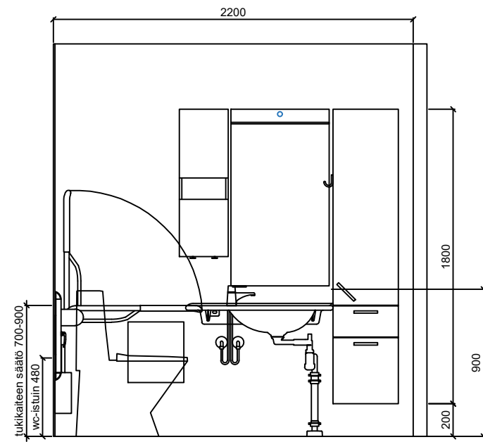
SEINÄKAAVIO A Gaius Sense 2XL
