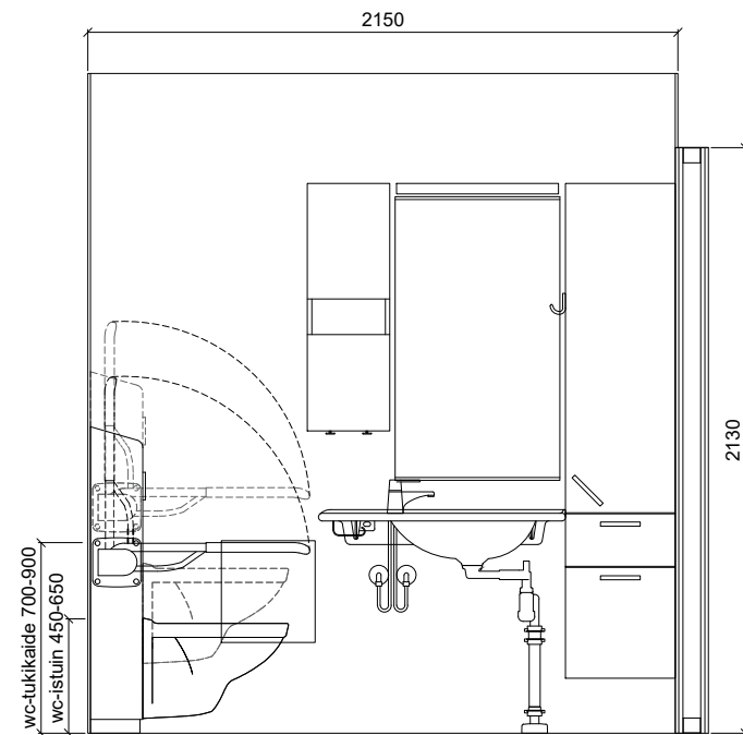
SEINÄKAAVIO A Gaius Original Sense XL, DUO
