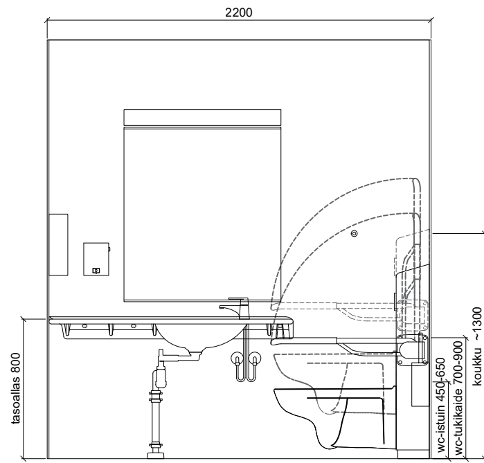
SEINÄKAAVIO A Gaius Public Babycare, DUO
