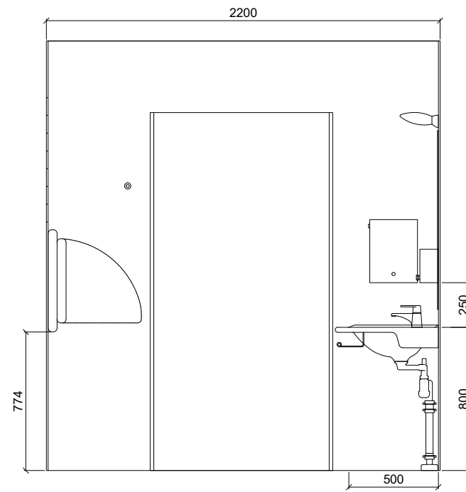
SEINÄKAAVIO B Gaius Public Babycare, DUO
